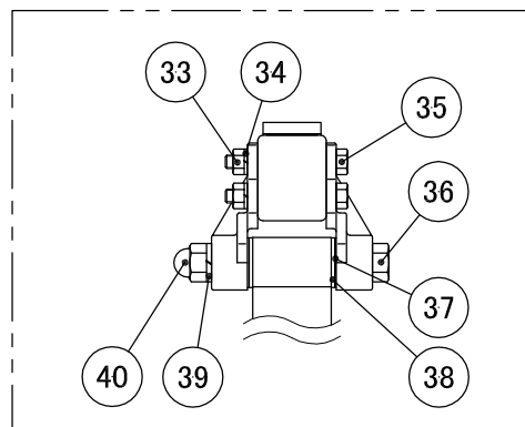
A部矢视图
